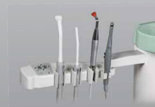
ПАНЕЛЬ АССИСТЕНТА С СЛЮНООТСОСОМ И ПЫЛЕСОСОМ (МОДЕЛЬ 300) И С ДВУМЯ ДОПОЛНИТЕЛЬНЫМИ ОПЦИЯМИ НА ВЫБОР (ШПРИЦ, ПОЛИМЕРИЗАЦИОННАЯ ЛАМПА, ИНТРАОРАЛЬНАЯ КАМЕРА) С ПЛЕНЧОЙ ПАНЕЛЬЮ УПРАВЛЕНИЯ ДЛЯ АССИСТЕНТА
